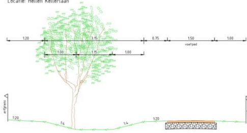
Dwarsprofiel 2-2
