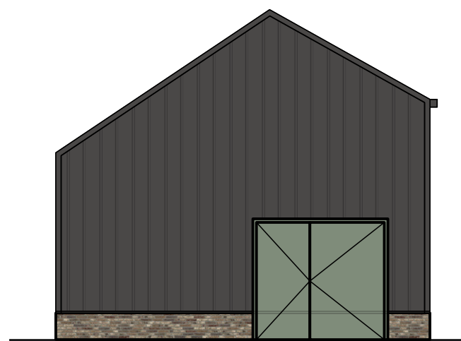
Kopgevel garage kavel 1 1:100
