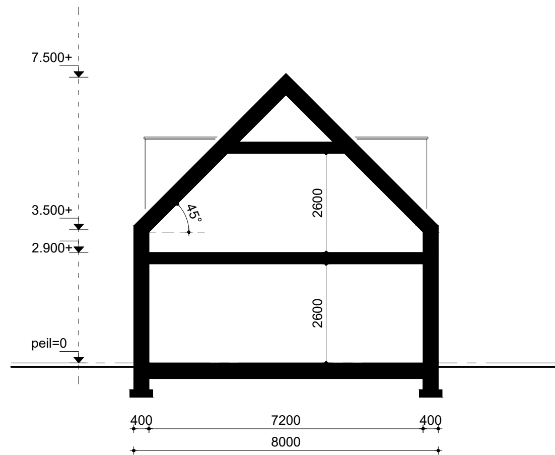
doorsnede Type 2 1:100
