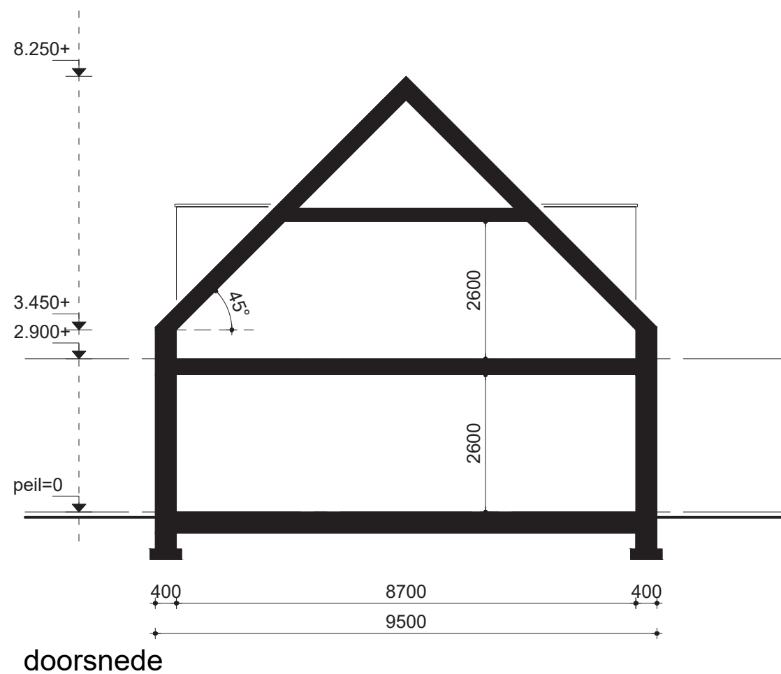
Type 1 1:100
