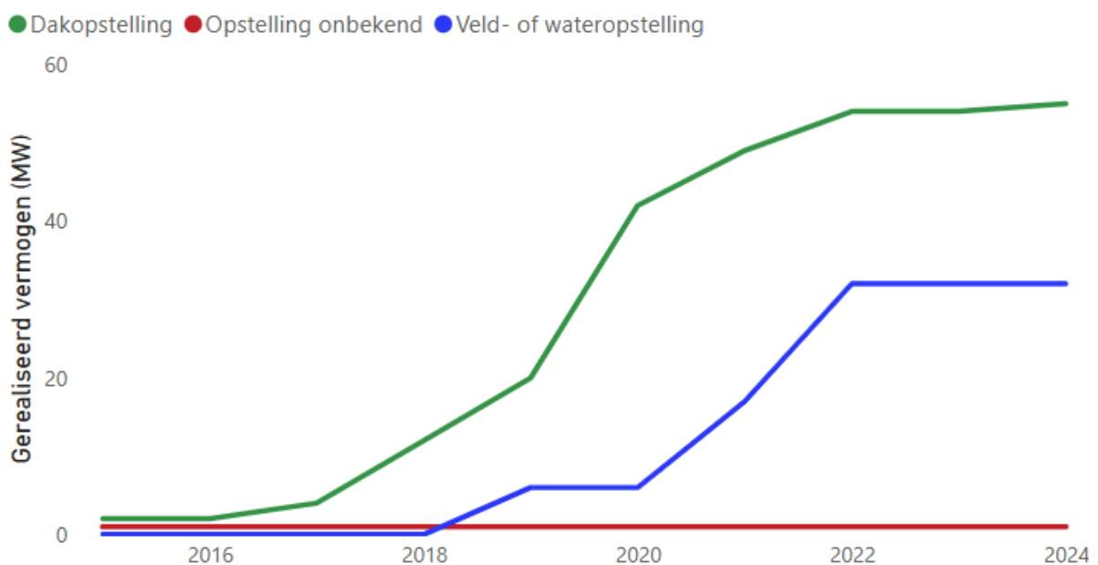
Figuur 9 Gerealiseerd vermogen zon in de RES-regio Amersfoort
