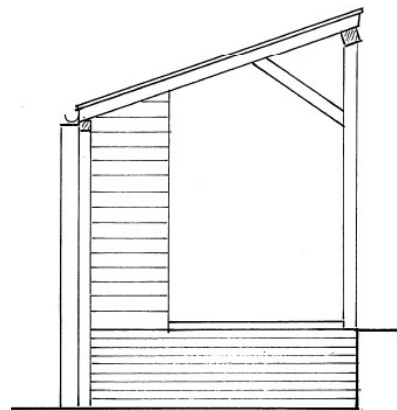
Doorsnede buitenkast
