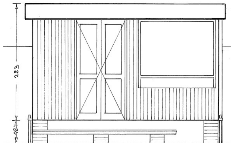
Aanzicht schafteket/schuur
