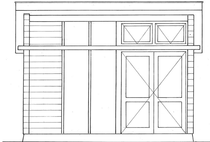
Aanzicht orangeriegebouwtje
